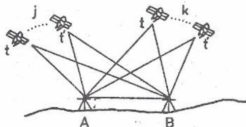
Obr. 2.25: GPS meranie pri tvorbe trojnásobných diferencií. (Zdroj: Sedlák, 2012).
