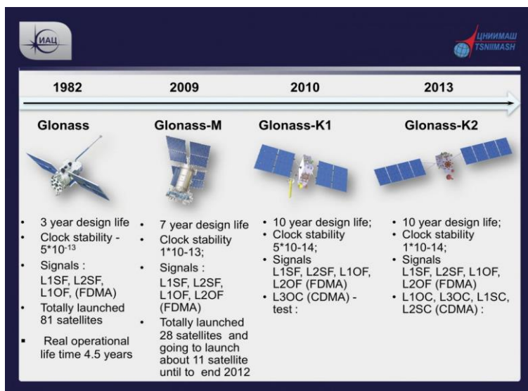
Obr. 2.37: Prehľad satelitov GLONASS. (Zdroj: Procházka, 2017).
