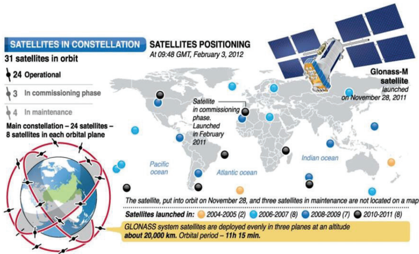
Obr. 2.38: Konštelácia satelitov GLONASS-M 3. februára 2012 o 09:48 GMT. (Zdroj: GLONASS navigation ..., 2012).
