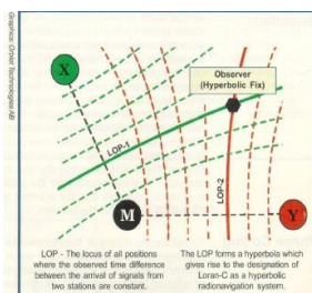
Obr. 1.10: Princíp činnosti a navigácie LORAN-C pre letectvo. (Zdroj: LORAN-C ... 2012; 1959 – LORAN C ... , 2017; upravené autorom).
