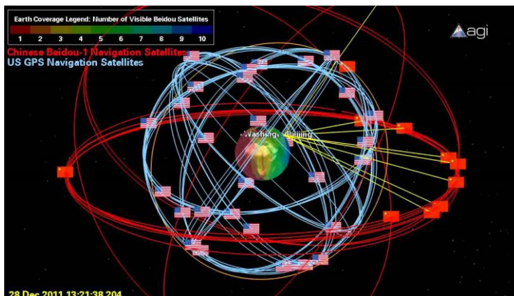
Obr. 2.52: Architektúra GPS a BeiDou-1. (Zdroj: China poised to orbit pair ..., 2018).
