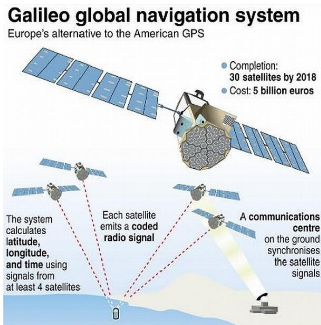
Obr. 2.42: Princíp satelitného navigačného systému Galileo. (Zdroj: Galileo, The new ..., 2017).
