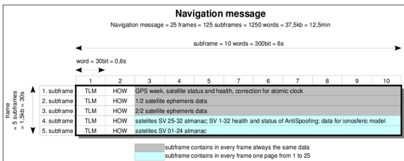
Obr. 2.13: Rôzne schematické znázornenia navigačnej správy GPS. (Zdroj: Why do GPS ..., 2017; Soubor:Navigation message ..., 2008).
