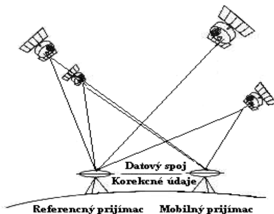
Obr. 2.17: Lokalizácia polohy pomocou GPS. (Zdroj: Sedlák, 2012).
