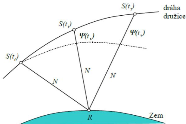
Obr. 2.22: Relatívne (fázové) GPS meranie so zmenami dráh satelitu. (Zdroj: Pisca, 2005).
