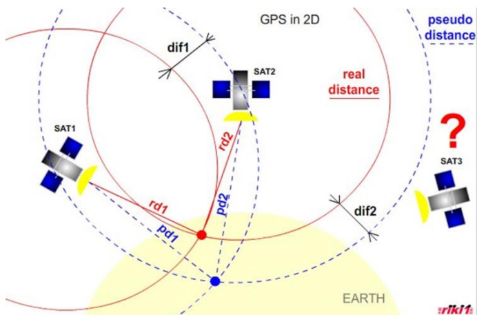
Obr. 2.20: Názorný príklad: Skutočná vzdialenosť a pseudovzdialenosť medzi satelitom a prijímačom GPS. (Zdroj: Prečo GPS ..., 2019).
