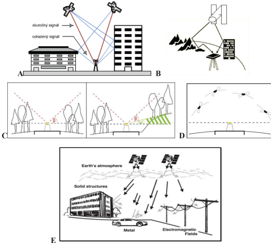
Obr. 2.34: Viaccestné, odrazené signály od budov (A) terénu, kovových objektov, elektromagnetického poľa (B) (E) a porastu (C); voľný priestor nad anténou (D). (Zdroj: Hodoň, 2010, upravené autorom).
