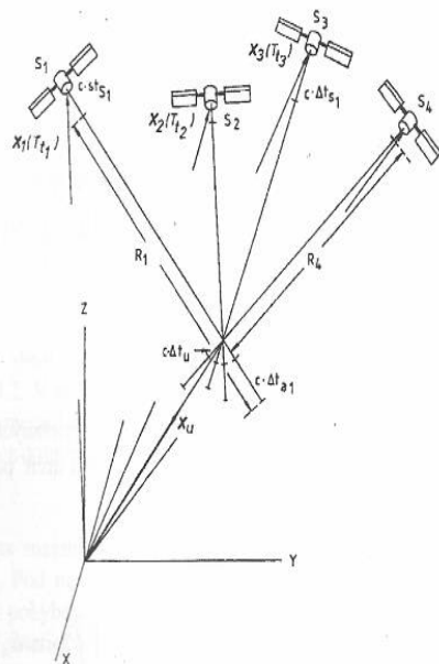
Obr. 2.21: Absolútne (časové, kódové) GPS meranie. (Zdroj: Sedlák, 2012).
