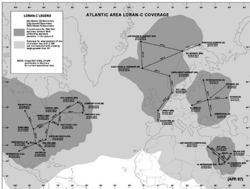
Obr. 1.12: Pokrytie atlantickej a pacifickej oblasti signálmi systému LORAN-C. (Zdroj: Government killing ... , 2010).
