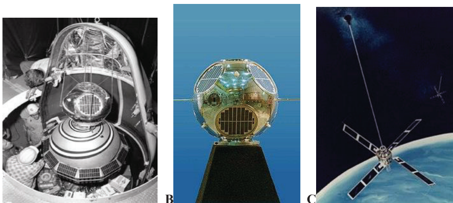
Obr. 1.14: TRANSIT 2A so satelitom GRAB 1 na vrchole počas prípravy na štartovanie (A); model satelitu GRAB v Národnom kryptologickom múzeu, USA (B); operačný satelit TRANSITu (C). (Zdroj: Transit (satellite), 2019; Galactic Radiation ... , 2019).
