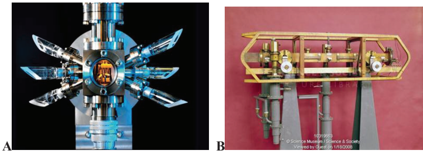
Obr. 2.9: Atómové hodiny - súčasnosť (A); prvé atómové hodiny z roku 1955 (B). (Zdroj: Jak se měří ..., 2016; Wagner, 2019).
