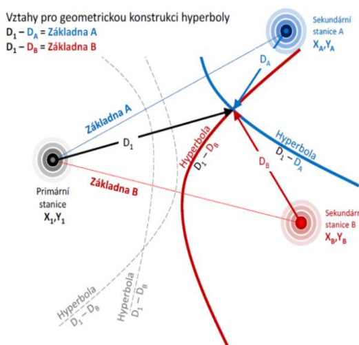
Obr. 1.11: Princíp hyperbolickej navigácie (časomerne hyperbolická metóda). (Zdroj: Vojtek, 2014).
