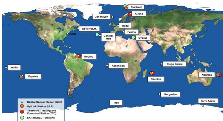
Obr. 2.49: Architektúra pozemného segmentu systému Galileo. (Zdroj: Galileo service ..., 2015).
