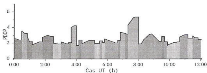
Obr. 2.31: Priebeh PDOP pre interval 12 hod.; B (latitude-zemepisná šírka) = 49°, L (longitude-zemepisná šírka = 20°, 15.11.2001, výškový filter 15°, 24 satelitov. (Zdroj: Sedlák, 2012).
