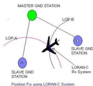
Obr. 1.10: Princíp činnosti a navigácie LORAN-C pre letectvo. (Zdroj: LORAN-C ... 2012; 1959 – LORAN C ... , 2017; upravené autorom).
