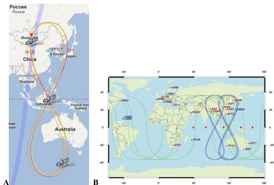
Obr. 2.53: Trajektórie navigačných satelitov BeiDou-2 (A); pozemné trajektórie pohybu satelitov BeiDou-2 s monitorovacími stanicami (B). (Zdroj: Beidou, 2019; Lou et al., 2014).
