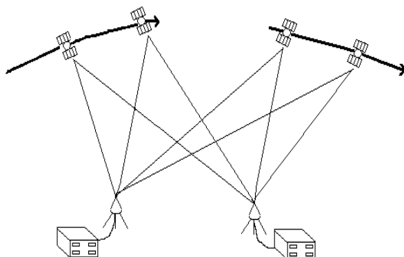
Obr. 2.27: Statická metoda. (Zdroj: Rapant, 2002).
