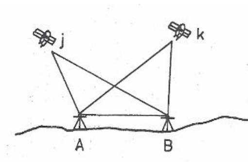
Obr. 2.24: GPS meranie pri tvorbe dvojnásobných diferencií. (Zdroj: Sedlák, 2012).
