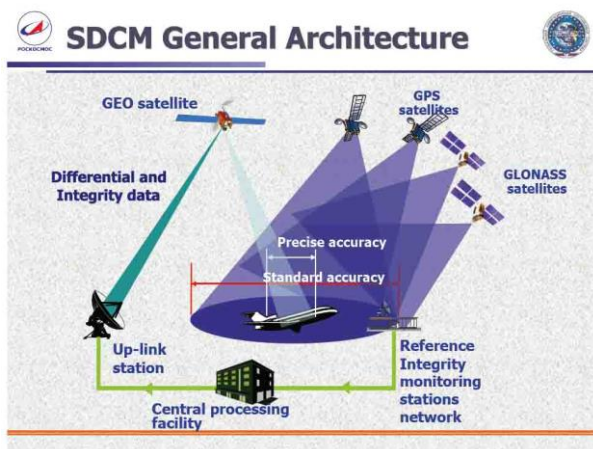
Obr. 3.11: Architektúra SDCM. (Zdroj: CIA, Pentagon trying ..., 2013).
