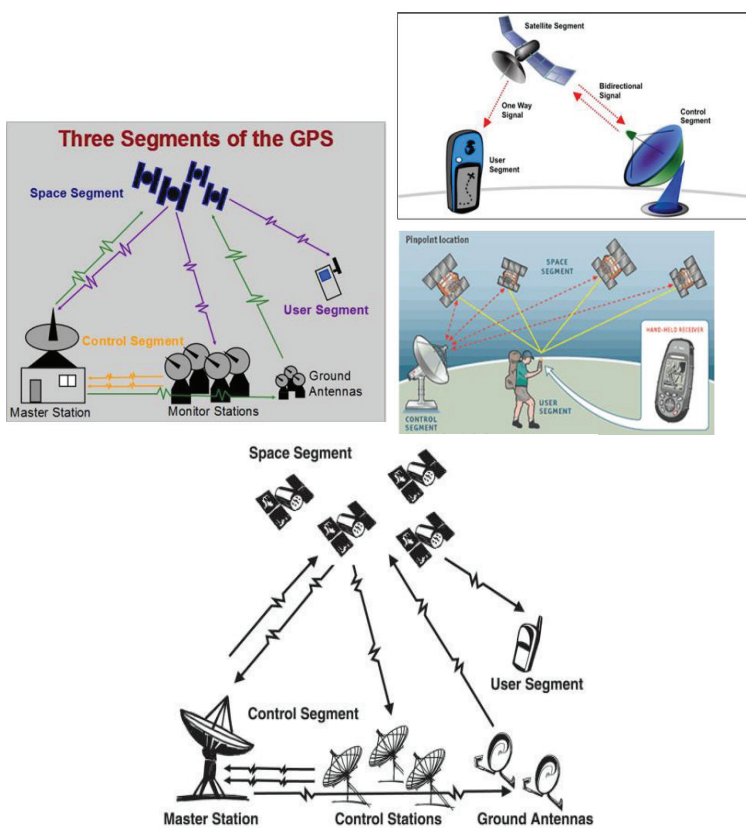
Obr. 2.4: Ukážky zobrazení a schém segmentov GPS. (Zdroj: Daryau, 2018; GPS, GIS and their uses, 2013).
