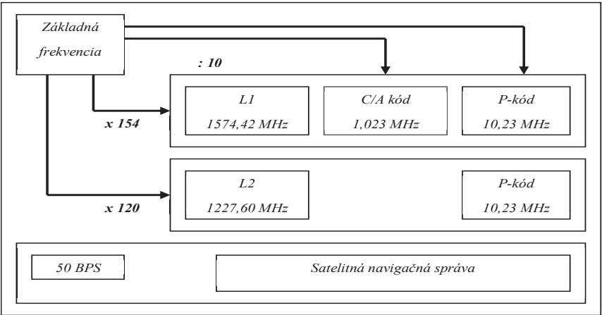
Obr. 2.12: Schéma odvodzovania frekvencií jednotlivých signálov GPS. (Zdroj: Sedlák a Lošonczi, 2011; Sedlák, 2012).
