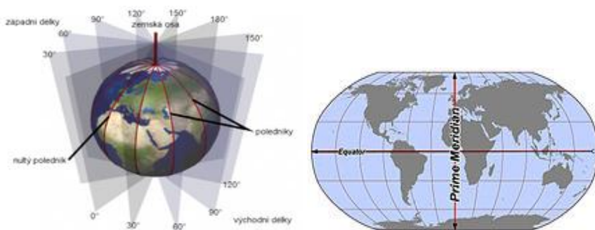
Obr. 1.7: Znáznornenie poludníkov a nultého (Greenwichského) poludníka. (Zdroj: Poludník, 2017; Greenwichský poludník, 2019).
