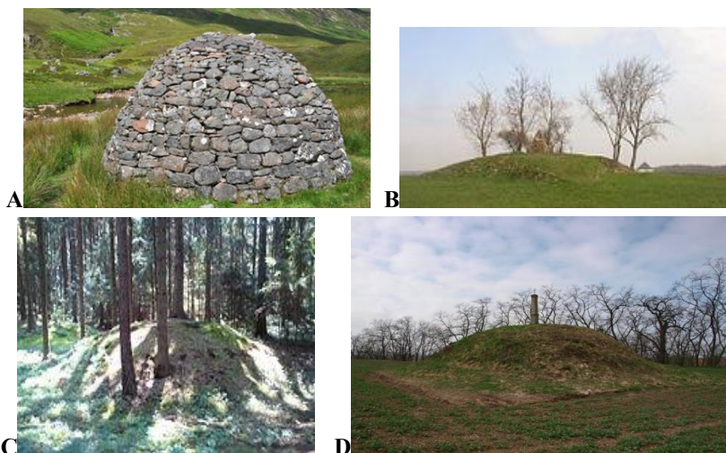
Obr. 1.1: Umelé orientačné body (objekty) v teréne: kamenný násyp (A); mohyla na Bielej hore v Prahe (B); mohyly na vrchu Baba u Vítína, okres České Budějovice (C); mohyla Homole - pravěká mohyla, Chotouň, Česká republika (D). (Zdroj: Cesty a památky, 2019; Mohyla, 2019; upravené autorom).
