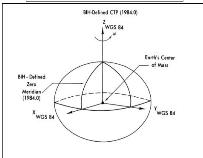
Obr. 2.35: WGS 84. (Zdroj: Svetový geodetický ..., 2018; World Geodetic ..., 2019).
