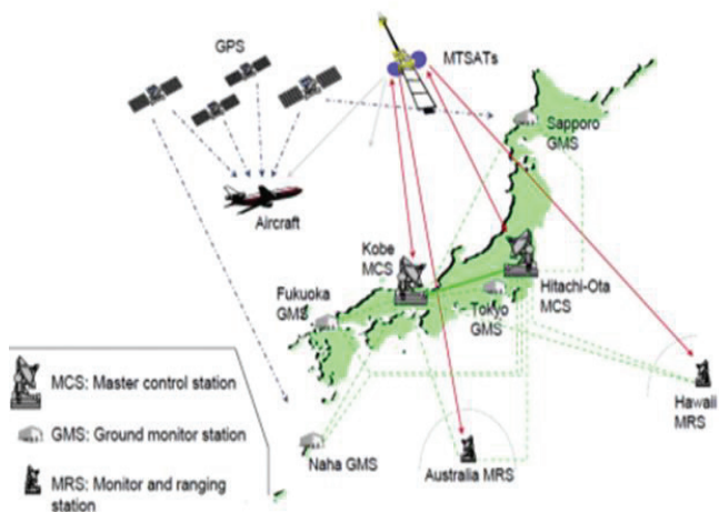
Obr. 3.9: Architektúra MSAS. (Zdroj: Satellite Navigation brings forth ..., 2019; upravené autorom; MSAS Architecture, 2019).
