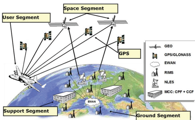
Obr. 3.1: Schéma architektúry SBAS. (Zdroj: SBAS Fundamentals, 2019).
