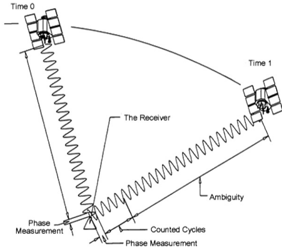
Obr. 2.23: Konceptia ambiguity pri fázovom meraní. (Zdroj: Pérez-Ruiz, 2012).
