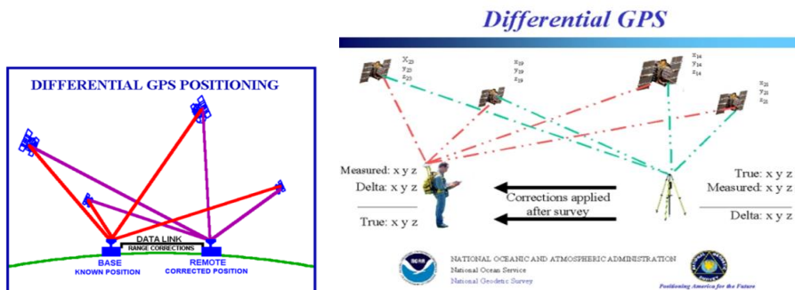
Obr. 2.26: Princíp určenia 3D polohy z diferenciálneho merania GPS. (Zdroj: GPS, 2002; Tecnología con ..., 2006; upravené autorom).
