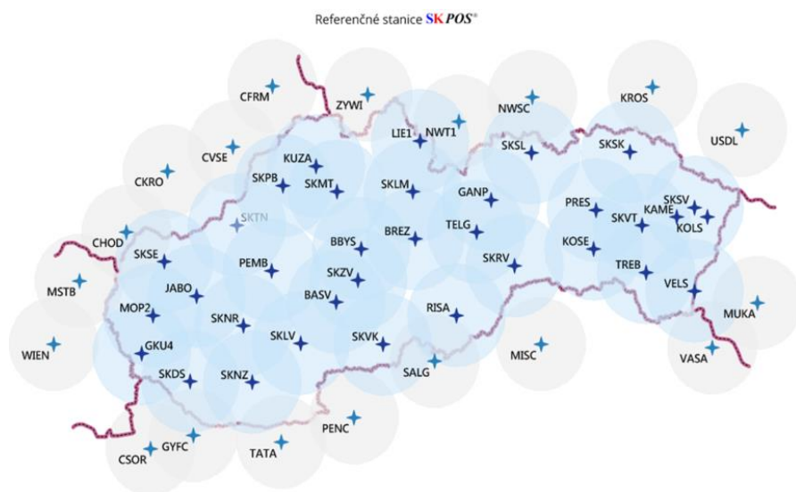
Obr. 2.2: Referenčné stanice SKPOS. (Zdroj: Slovenská priestorová ..., 2017).
