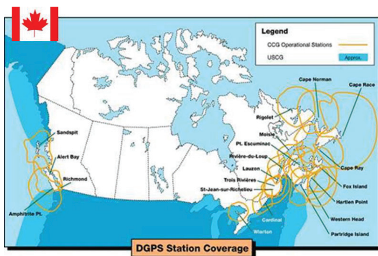
Obr. 3.13: Pokrytie Kanady službou DGPS z GPS-C/CWAAS . (Zdroj: Primer on GPS and DGPS, 2019; upravené autorom).
