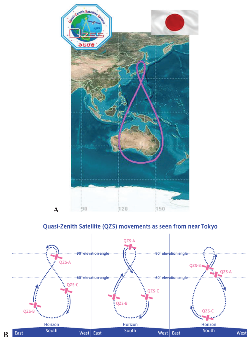
Obr. 3.4: QZSS (Japonsko) (A); orbity satelitov QZSS (B). (Zdroj: Quasi-Zenith ..., 2019a; upravené autorom; Quasi-Zenith ... , 2019b).
