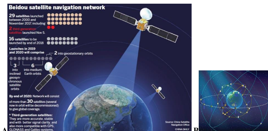
Obr. 2.50: Navigačný satelitný systém BeiDou (Compass); základné dáta (A); konštelácia satelitov (B). (Zdroj: China's BeiDou navigation ..., 2018; Beidou, 2019).
