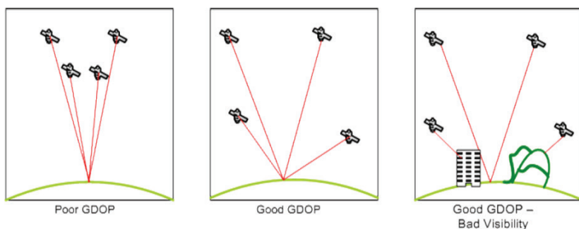
Obr. 2.30: Ukážky konfigurácie štyroch satelitov s rôznymi faktormi GDOP (geometrický faktor zníženia presnosti). (Zdroj: GPS Study ..., 2019).
