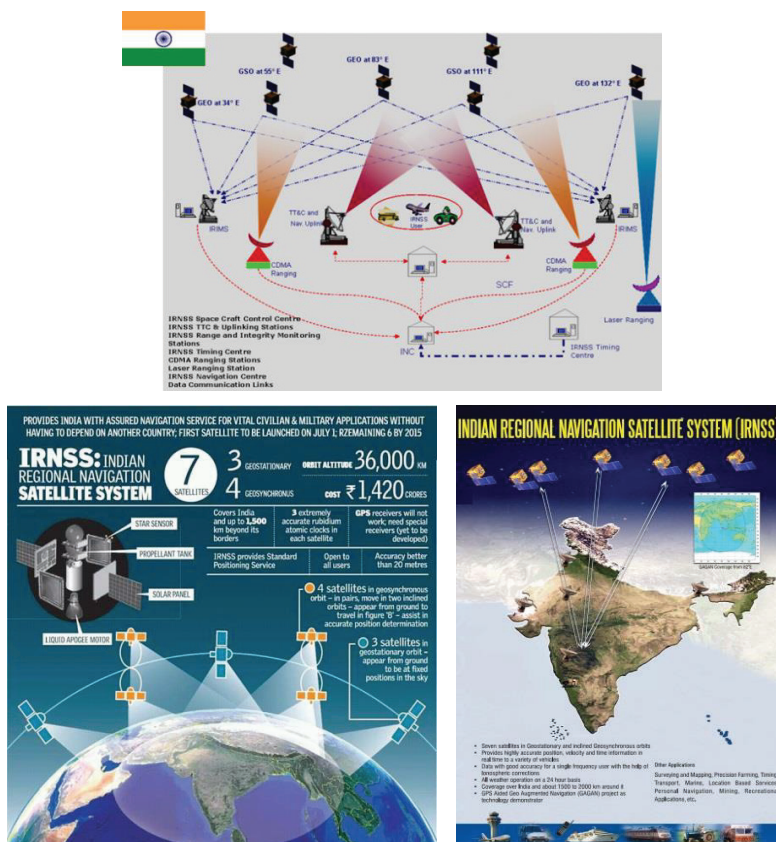
Obr. 3.5: Rôzne schémy architektúry IRNSS. (Zdroj: Vasantha Kumar, 2015; upravené autorom; IRNSS - Basic facts, 2016; Indian regional ..., 2013).
