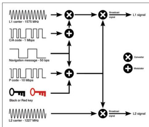
Obr. 2.11: Schéma modulácie signálu vysielaného satelitom GPS. (Zdroj: Drahovský, 2010).
