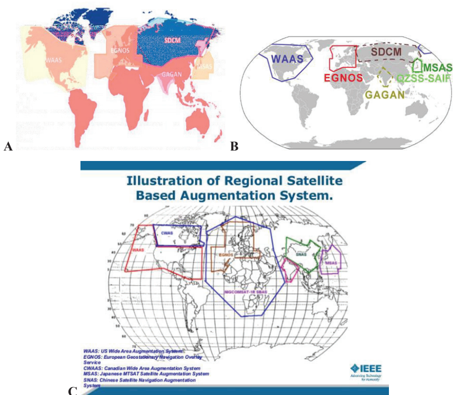
Obr. 3.2: Geografické rozmiestnenie a dosah niektorých SBAS v rôznych interpretáciách (A,B,C). (Zdroj: What is SBAS, 2019; GNSS augmentation, 2019; Salami, 2015).
