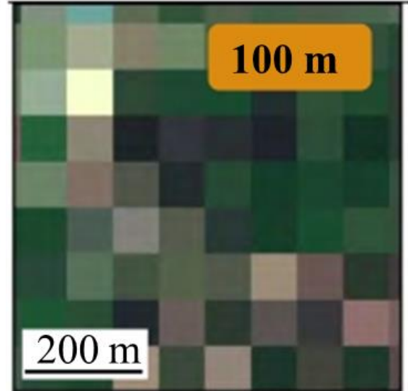
PROBA-V
