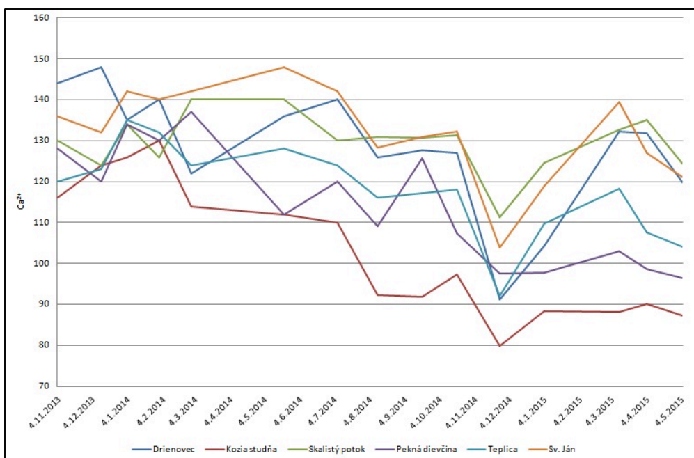
Fig. 6. Ca 2+ content
